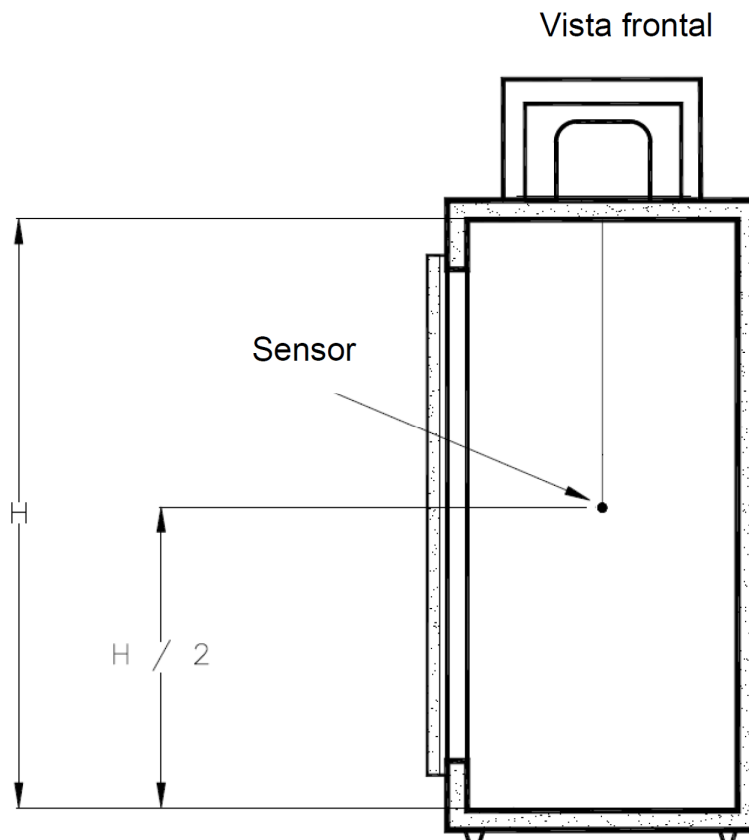
Figura E.18 - Colocación de sensor en conservador de hielo
