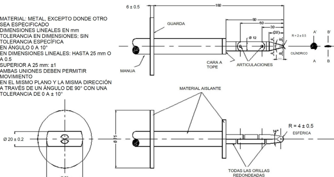
Figura A.1 - Dedo de prueba articulado
