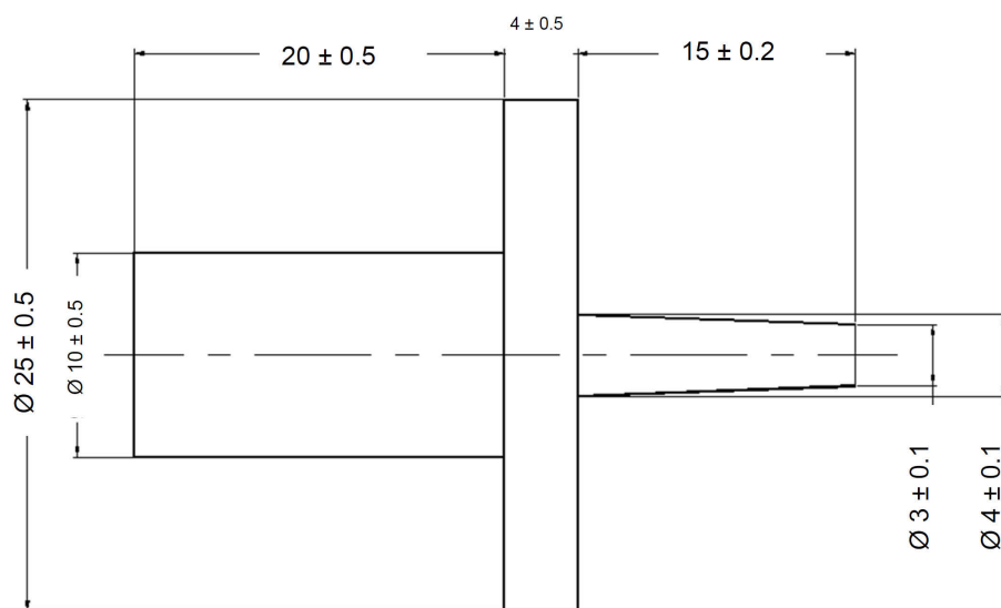
Figura A.2 - Aguja de prueba
