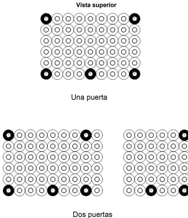
Figura E.12 - Colocación de sensores de prueba en enfriador horizontal con circulación forzada de aire vista superior
