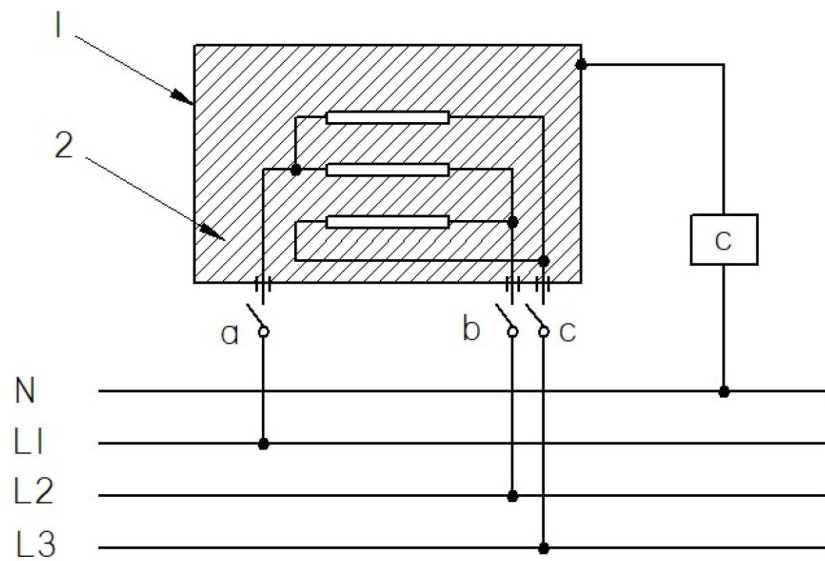
Figura A.6 - Aparatos de Clase II trifásicos
