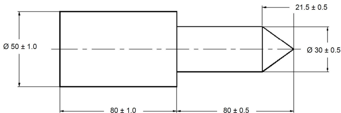
Figura A.3 - Probeta de prueba
