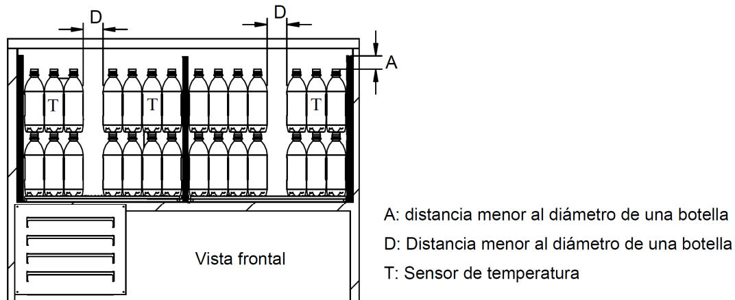
Figura E.13 - Colocación de sensores de prueba en enfriador horizontal de placa fría
