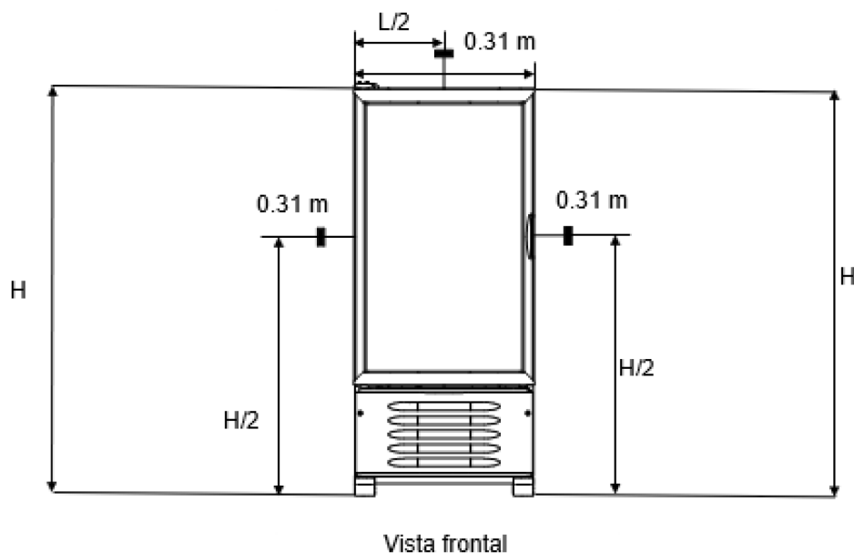
Figura D.1 - Colocación de los medidores
