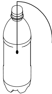
Figura E.4 - Colocación de sensor dentro de producto de prueba (PET o botella)
