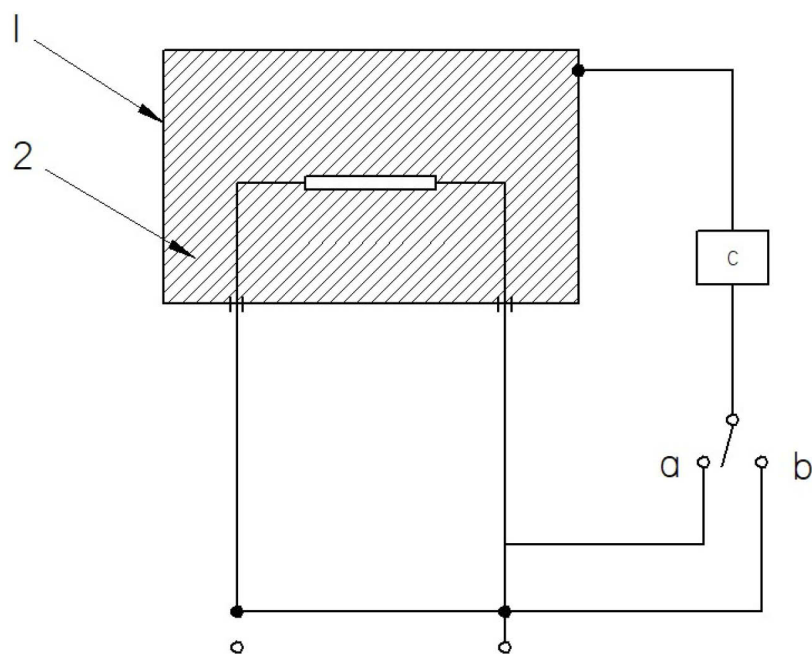
Figura A.4 - Diagrama para la medición de corriente de fuga a la temperatura de operación para aparatos
