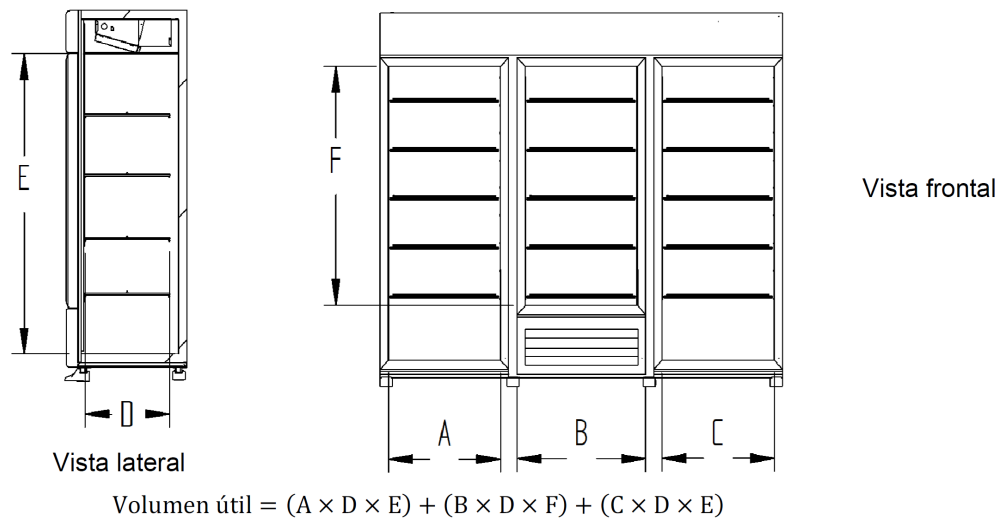
Figura C.6 - Cálculo del volumen útil de enfriadores y congeladores verticales unidad condensadora en el centro de gabinete
