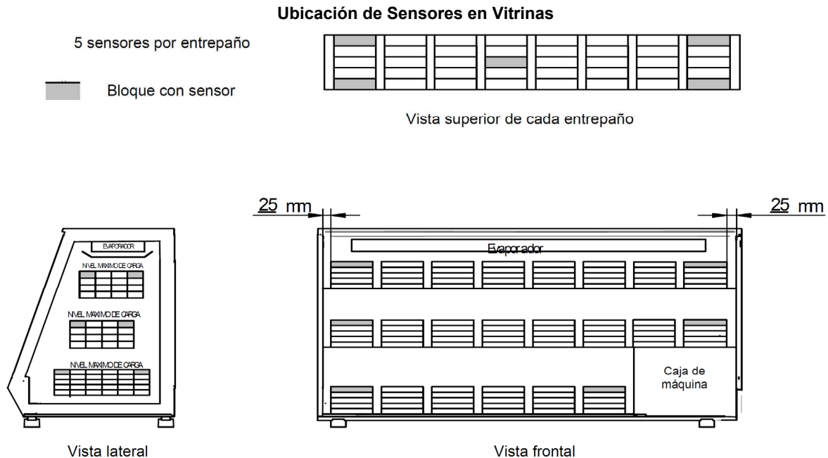
Figura E.17 - Colocación de bloque con sensor en vitrina refrigerada cerrada con puertas
