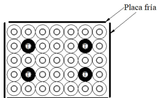
Figura E.14 - Colocación de sensores en enfriador horizontal de placa fría vista superior
