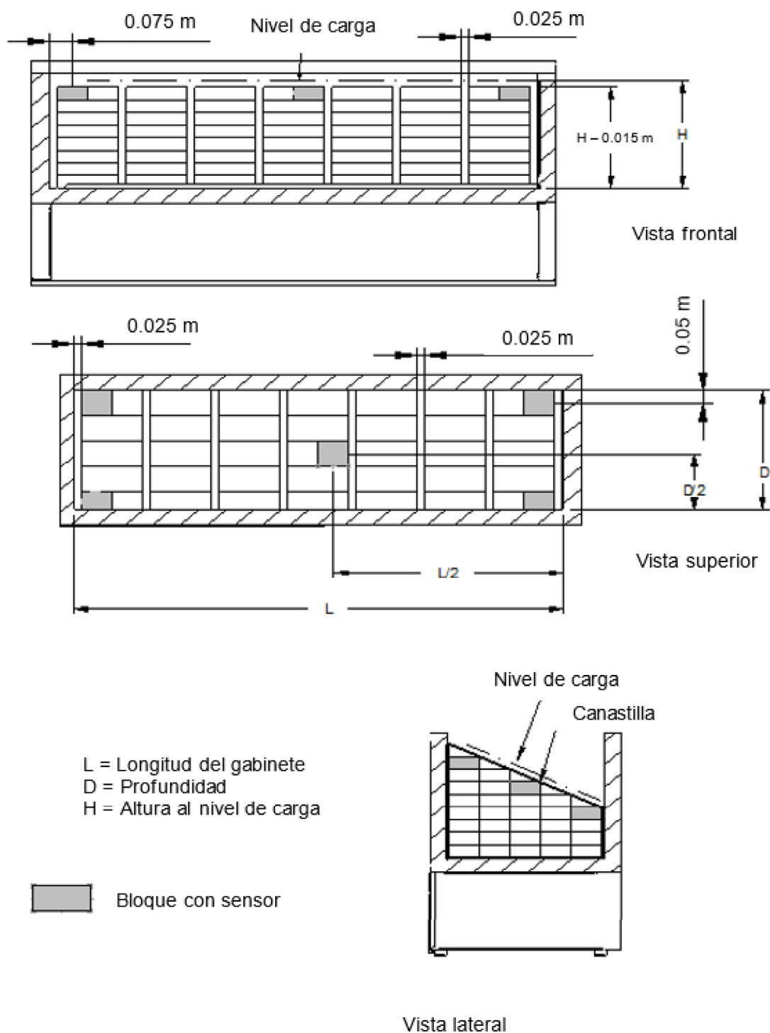
Figura E.16 - Colocación de sensor en congeladores horizontales
