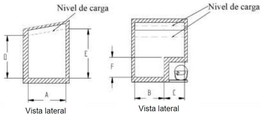
Figura C.3 - Cálculo del volumen útil de enfriadores y congeladores horizontales
