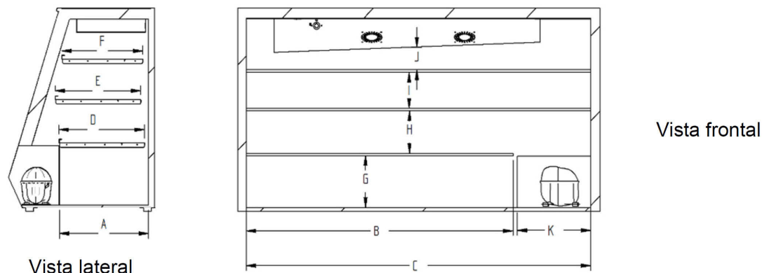
Figura C.8 - Cálculo de volumen útil de vitrina refrigerada cerrada con puertas (ejemplo 1)
