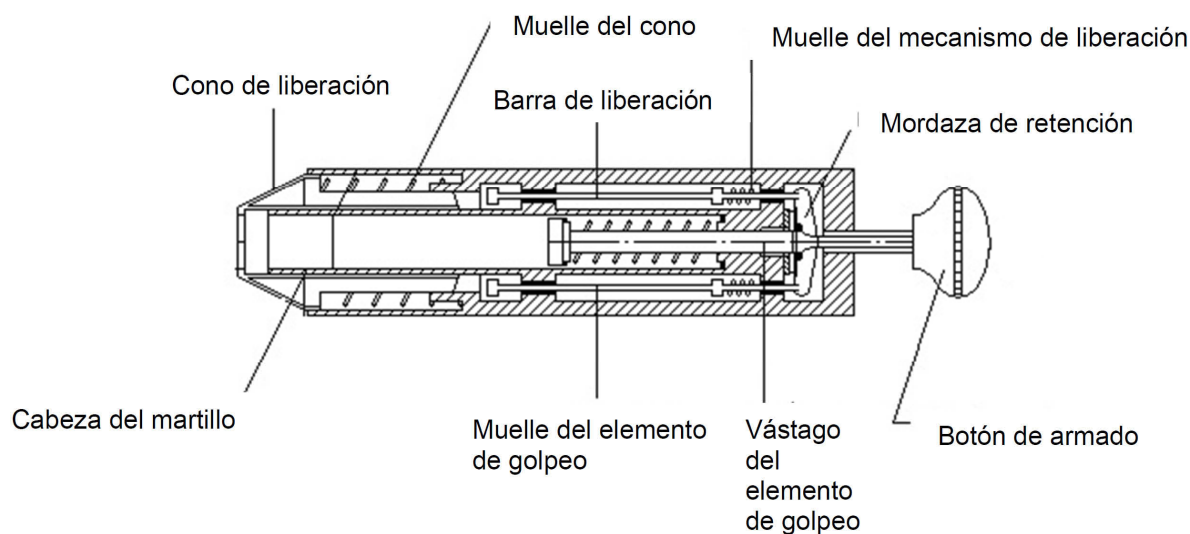
Figura A.8 – Equipo de prueba de martillo de resorte
