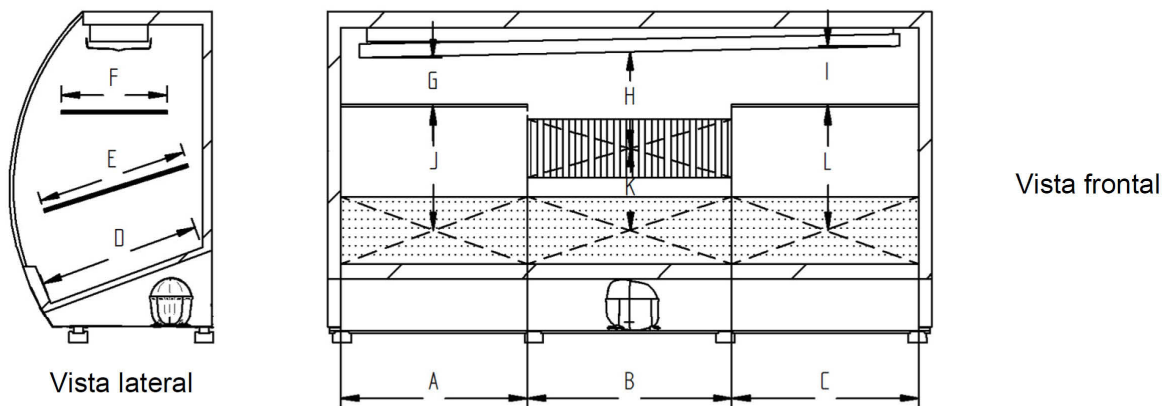
Figura C.10 - Cálculo de volumen Útil de Vitrina refrigerada cerrada con puertas y vidrio curvo
