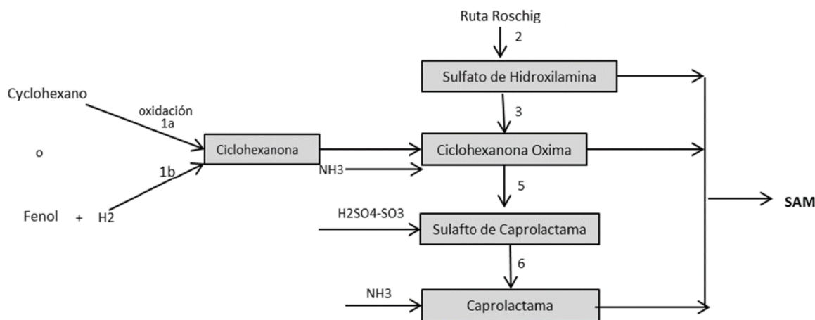
Diagrama 1. Proceso productivo del sulfato de amonio
